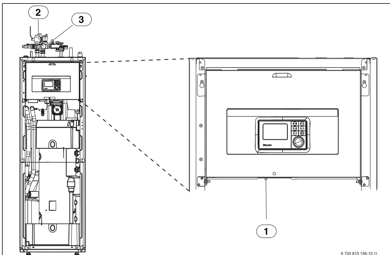
Bild 5 Inneenhet AirModule S / SS
