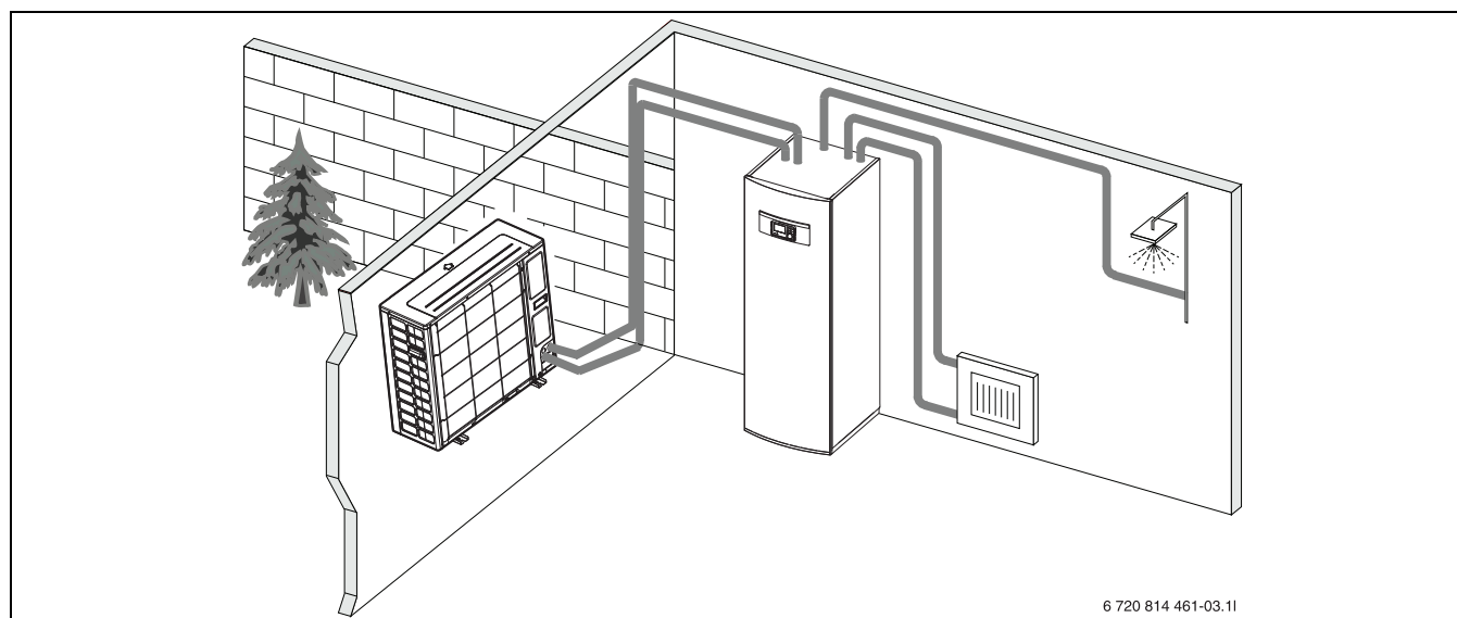
Bild 2 Uteenhet, inneenhet AirModuleS/SS med integrerad varmvattenberedare och eltilskott
