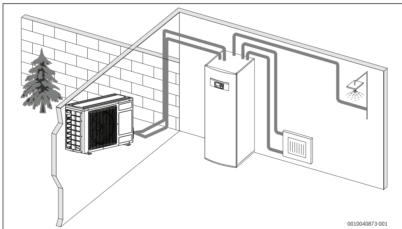
Bild 2 Värmepump för uteenhet, inneenhet AirModule Split med integrerad varmvattenberedare och elektriskt värmeelement
