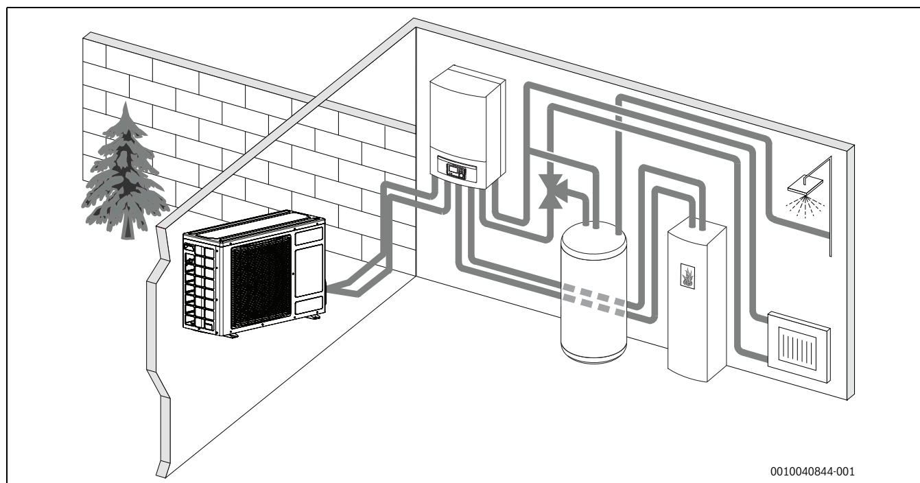
Bild 2 Värmepump för uteenhet, inneenhet AirBox Split S utan eltilskott, extern varmvattenberedare och extern extra värmekälla
