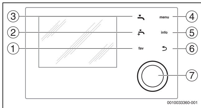
Bild 5 Manöverelement
